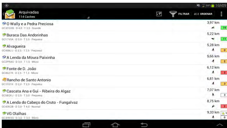
Figura 6. C:Geo, arquivo
