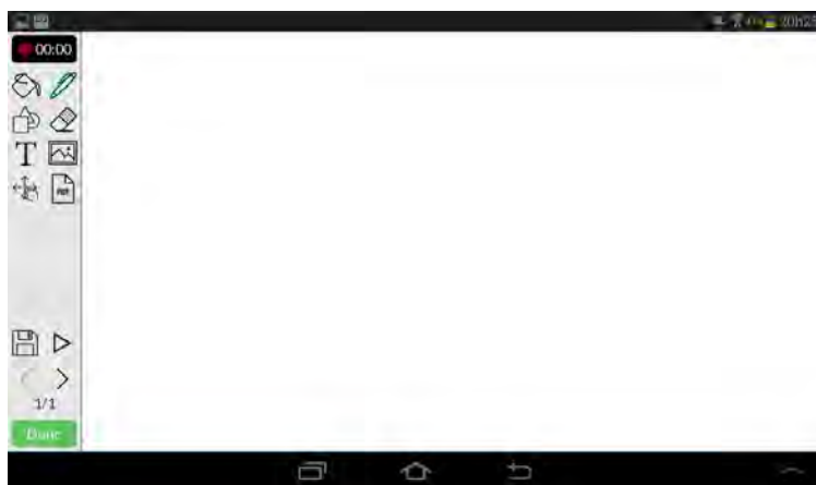
Figura 8. Nova gravação
