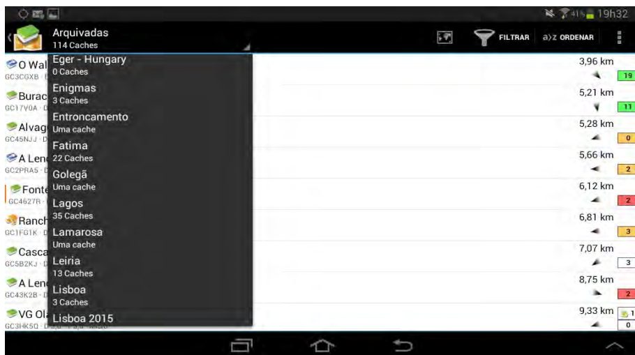
Figura 7. C:Geo, listas
